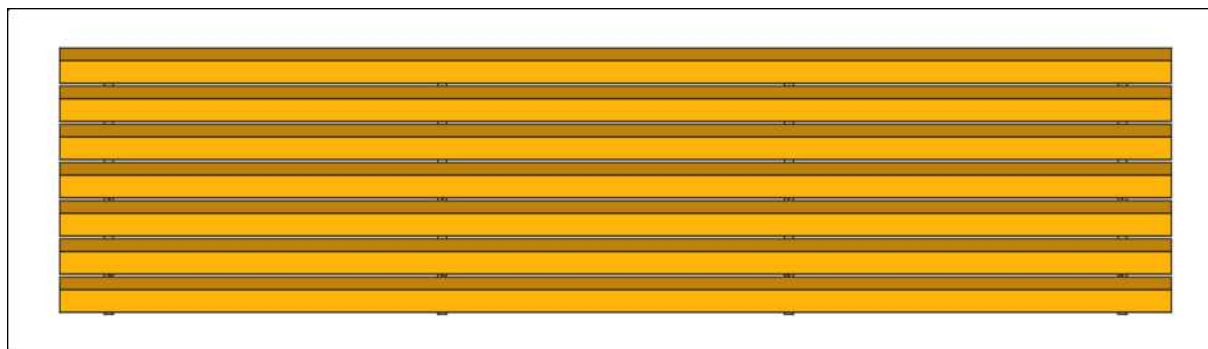
Abb. 5: Modul mit 7 Leisten auf 60 cm Elementhöhe; Abstand B = 8,6 cm
