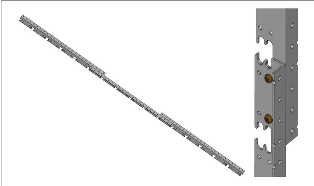
Abb. 22: Verlängerte BRIGX Winkel
