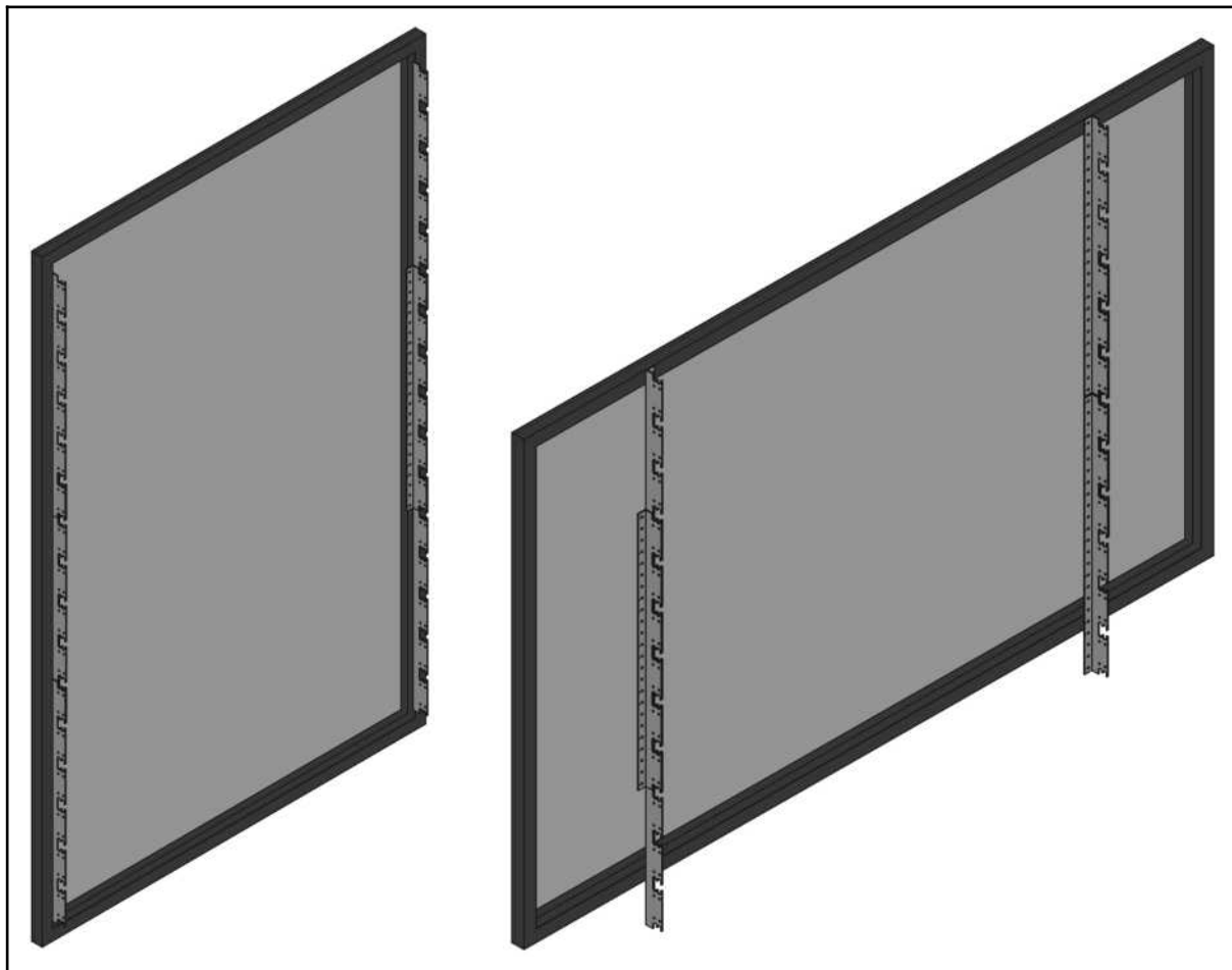
Abb. 23: Verlängerte BRIGX Winkel an PV-Modulen im Hoch- und Querformat
