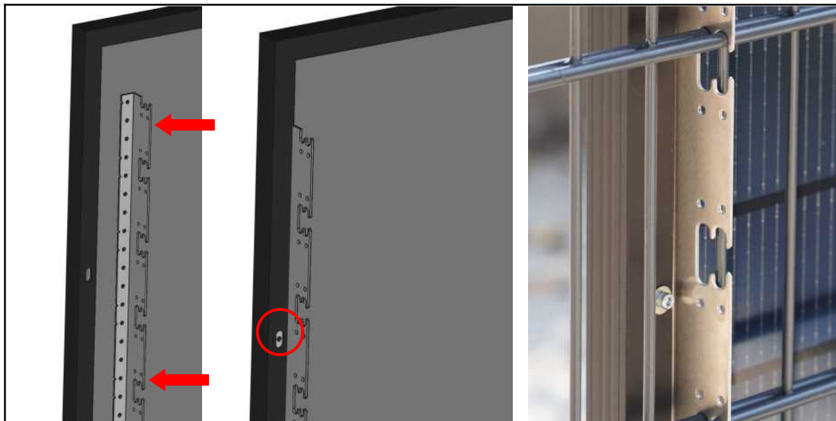
Abb. 24: Einlegen und Montieren der Winkel
