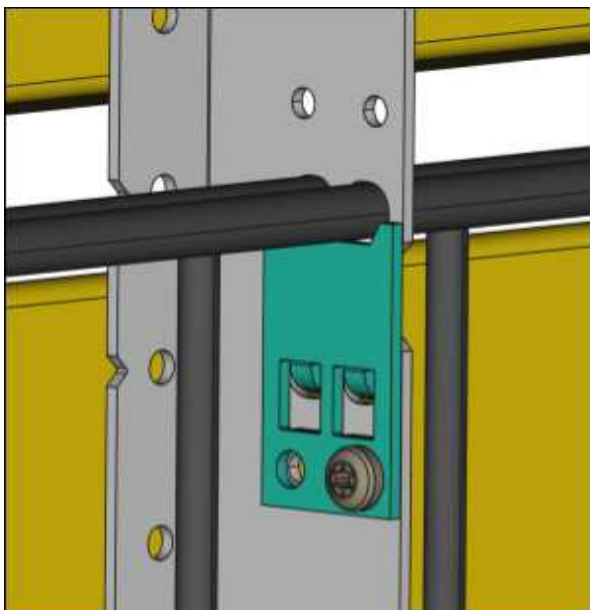
Abb. 12: Schraube in rechter Bohrung
