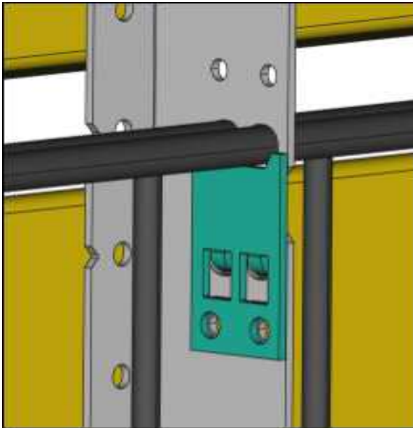
Abb. 10: Aushebesicherung in Winkellinnenseite
