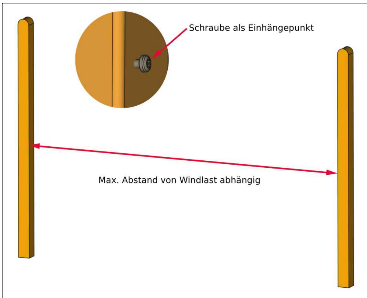
Abb. 16: Pfostenabstand und Einhängpunkt
