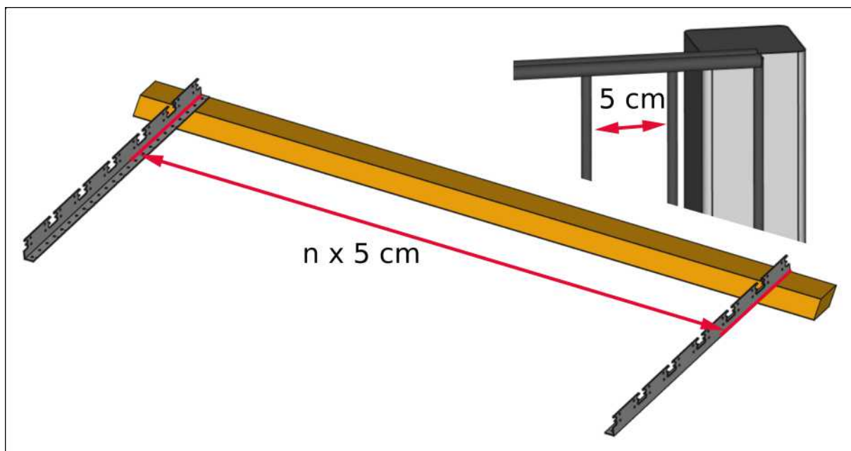
Abb. 2: Ermittlung der Abschlusswinkelposition auf einem Sichtschutzelement
