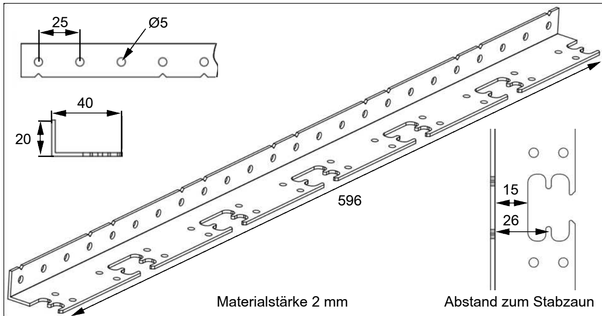
Abb. 28: Produktabmessungen BRIGX Winkel
