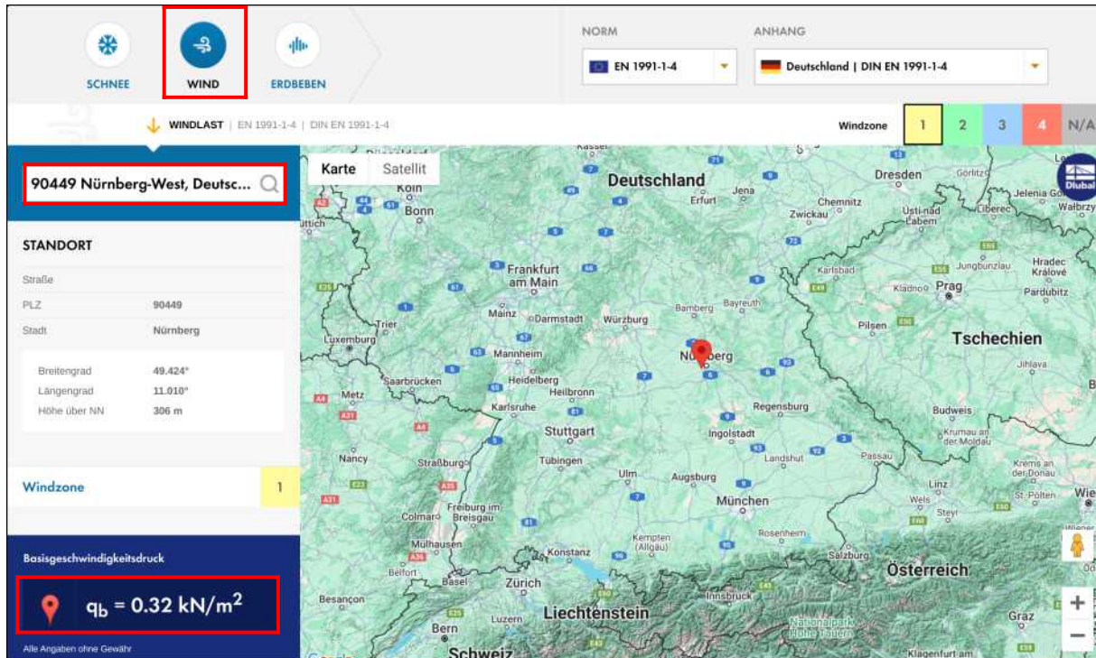
Abb. 21: Ermittlung des Basisgeschwindigkeitsdrucks mit www.dlubal.com
