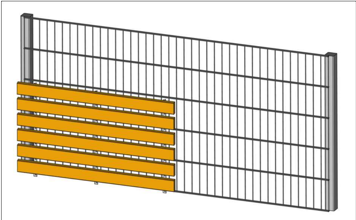
Abb. 9: Setzen des ersten Elements
