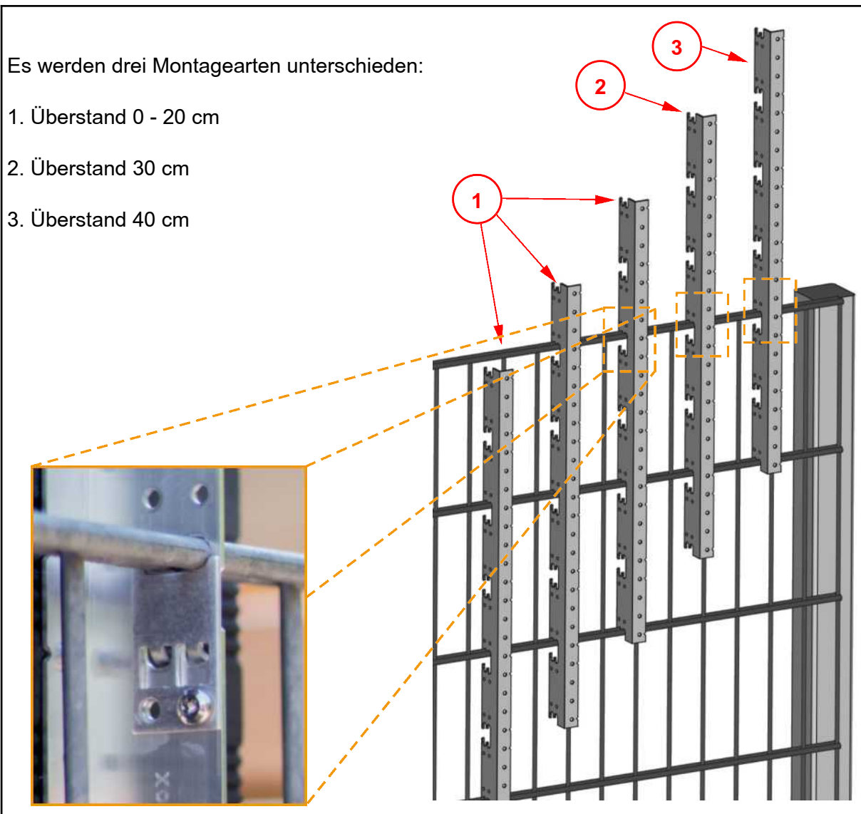
Abb. 8: Überstandsvarianten und Position der BRIGX Aushebesicherung am Doppelstabzaun
