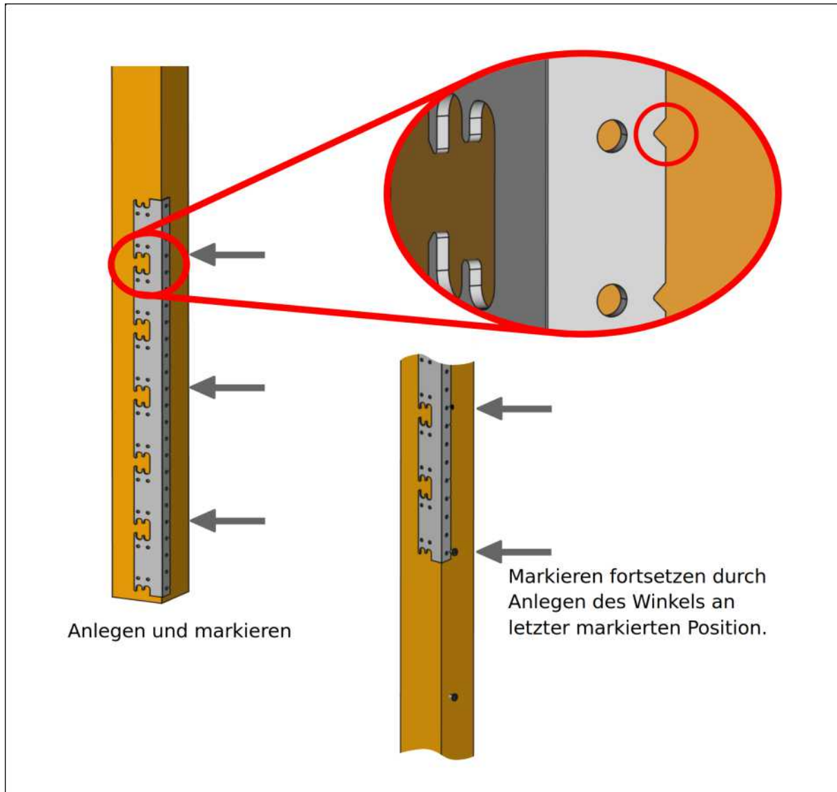
Abb. 17: Vorgehensweise bei Herstellung der Einhängpunkte am Pfosten
