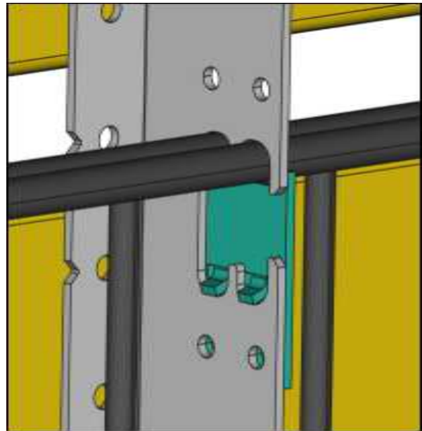
Abb. 11: Aushebesicherung in Winkelaußenseite
