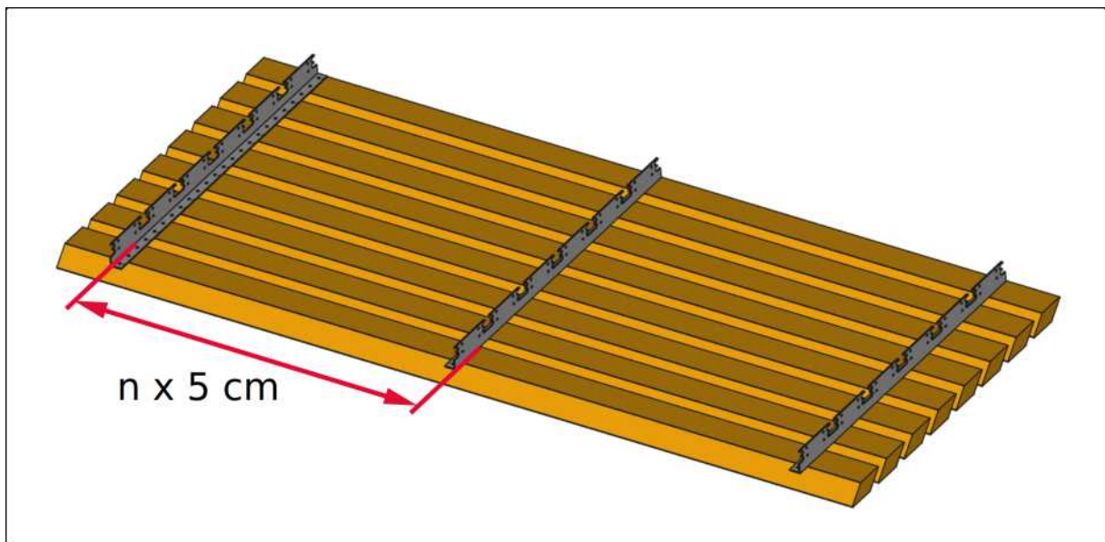
Abb. 7: Ermittlung der Abstände der Zwischenwinkel
