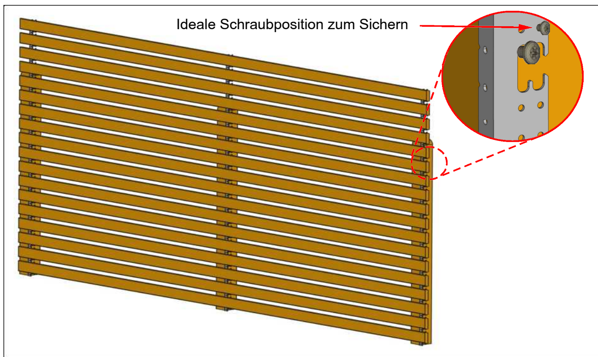
Abb. 19: Schraubposition zum sichern gegen Ausheben an eingehängtem Pfostenelement mit Überstand
