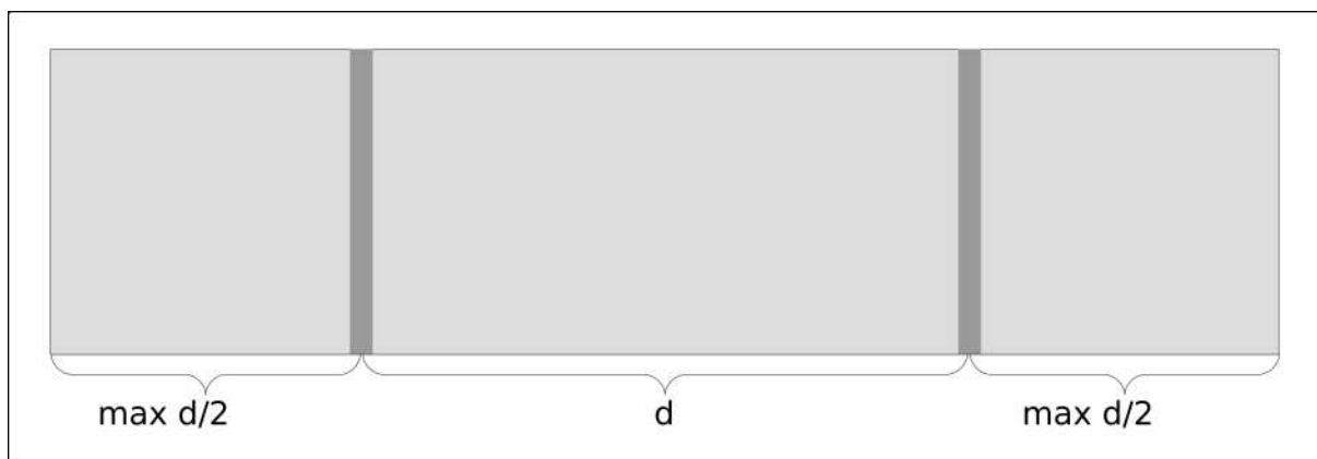
Abb. 20: Mögliche Verteilung der BRIGX Winkel auf einem Element
