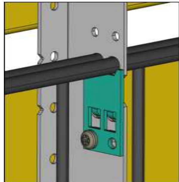
Abb. 13: Schraube in linker Bohrung
