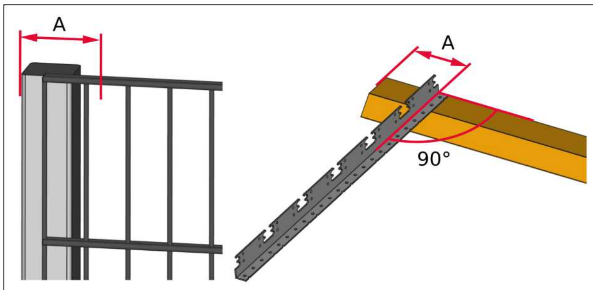
Abb. 1: Übertragen der Anfangsposition des ersten BRIGX-Winkels auf ein Sichtschutzelement
